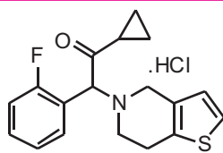
Prasugrel Desoxo Impurity
